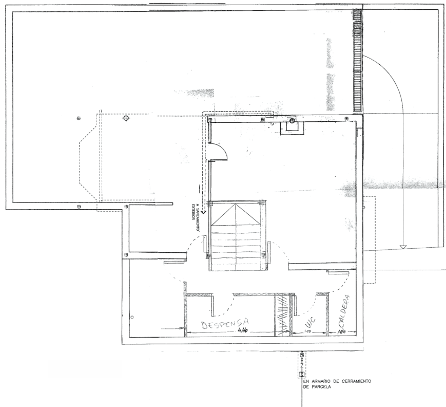
PLANTA SÓTANO
