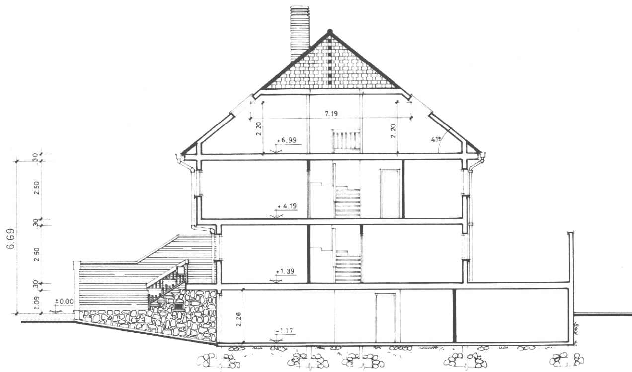
SECCION 2-2
