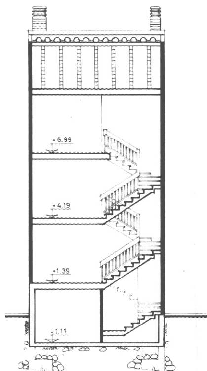
SECCION 1-1
