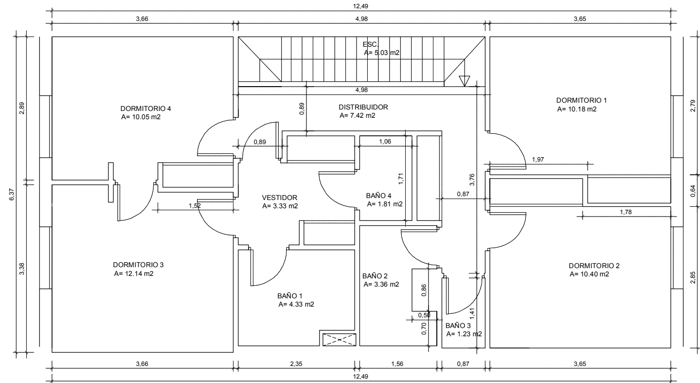
PLANTA PRIMERA
