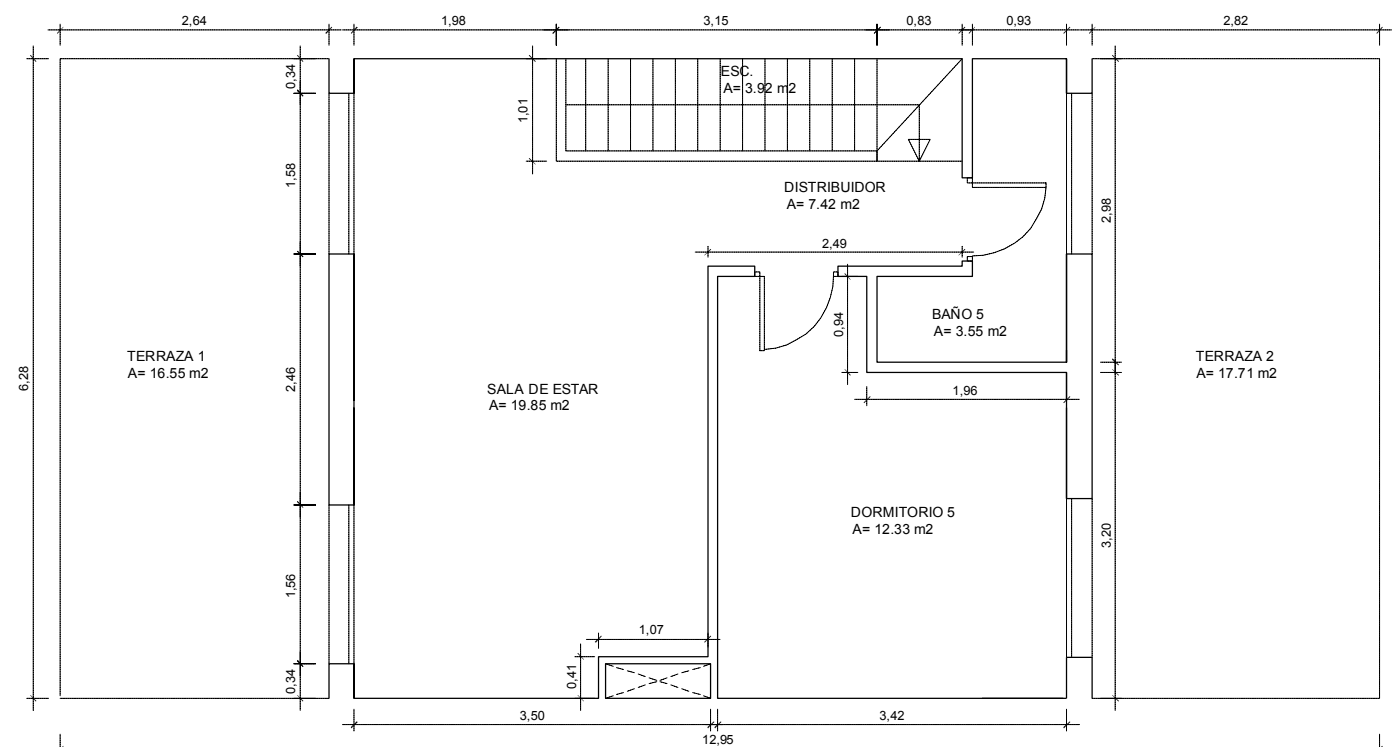
PLANTA SEGUNDA
