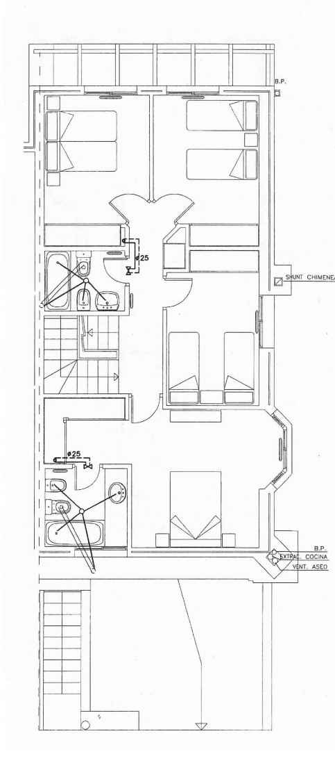
PLANTA PRIMERA
