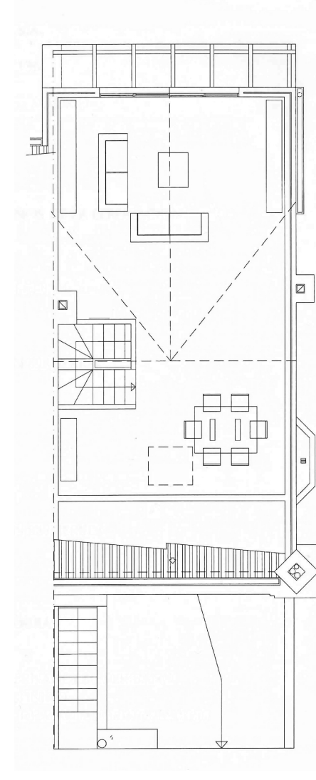
PLANTA ÁTICO
