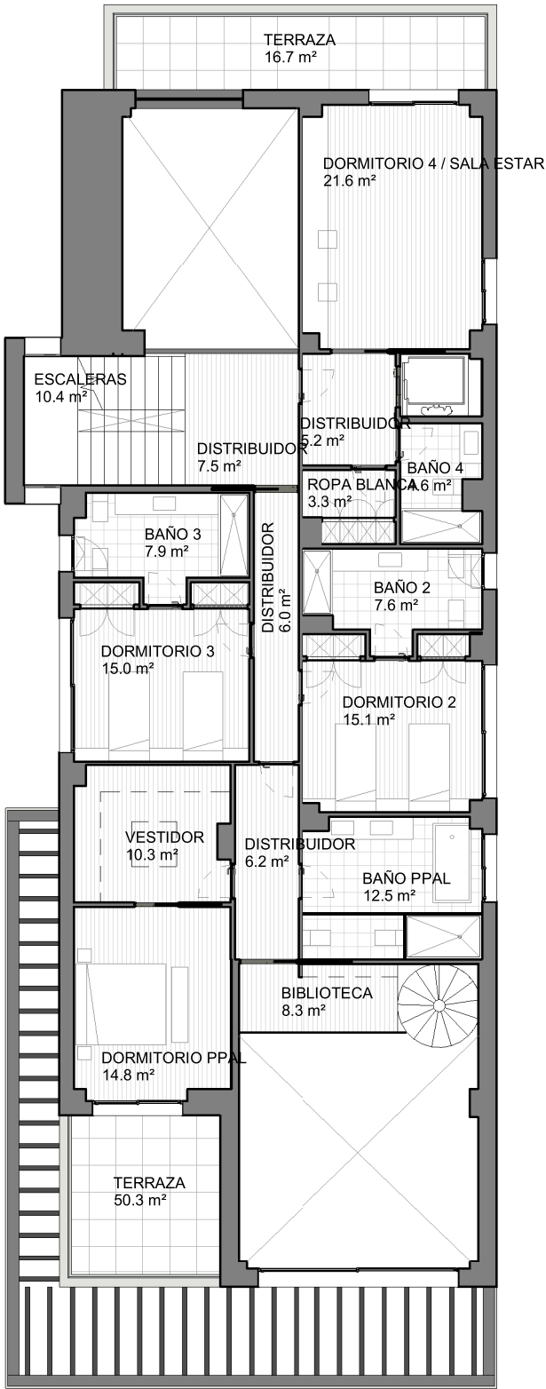
PLANTA PRIMERA 1 : 150
