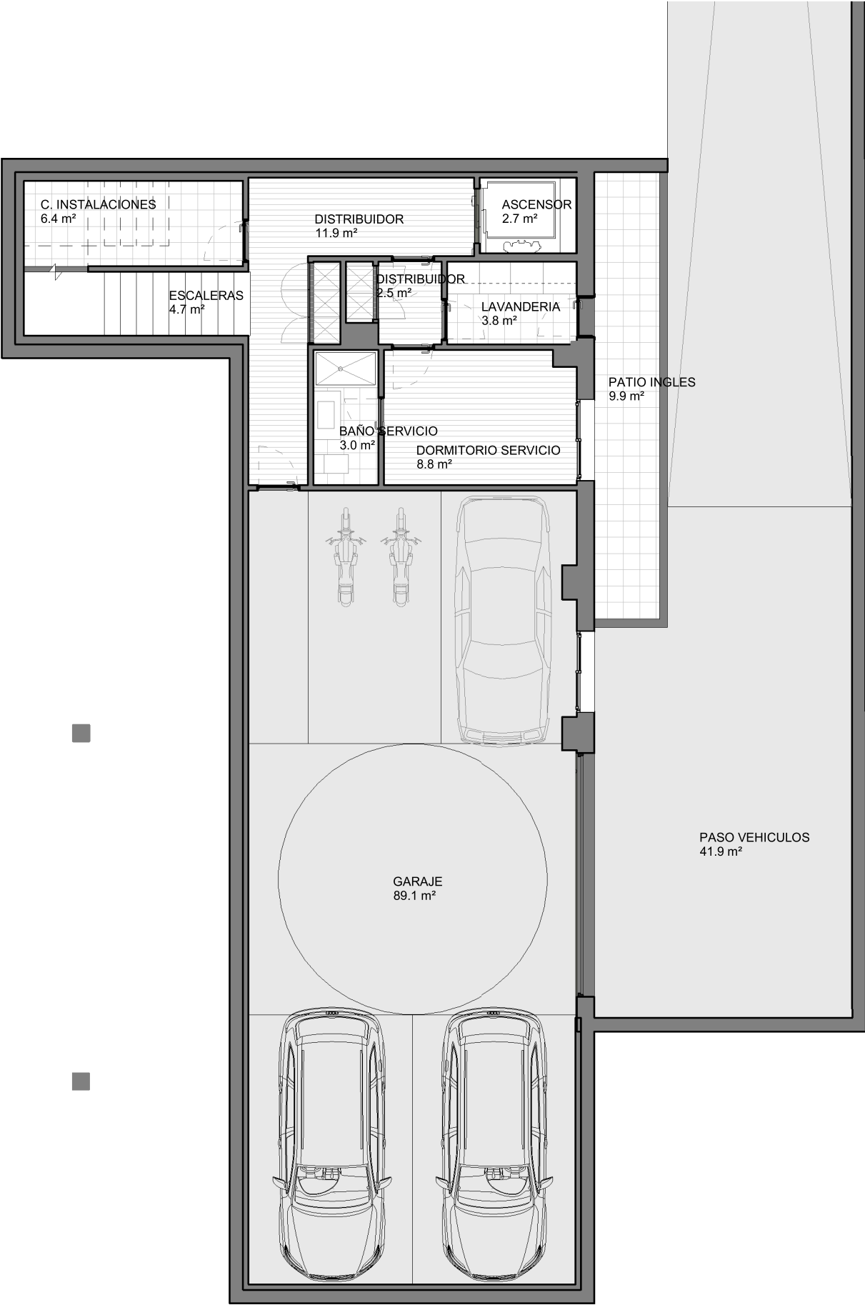
PLANTA SOTANO 1 : 100
