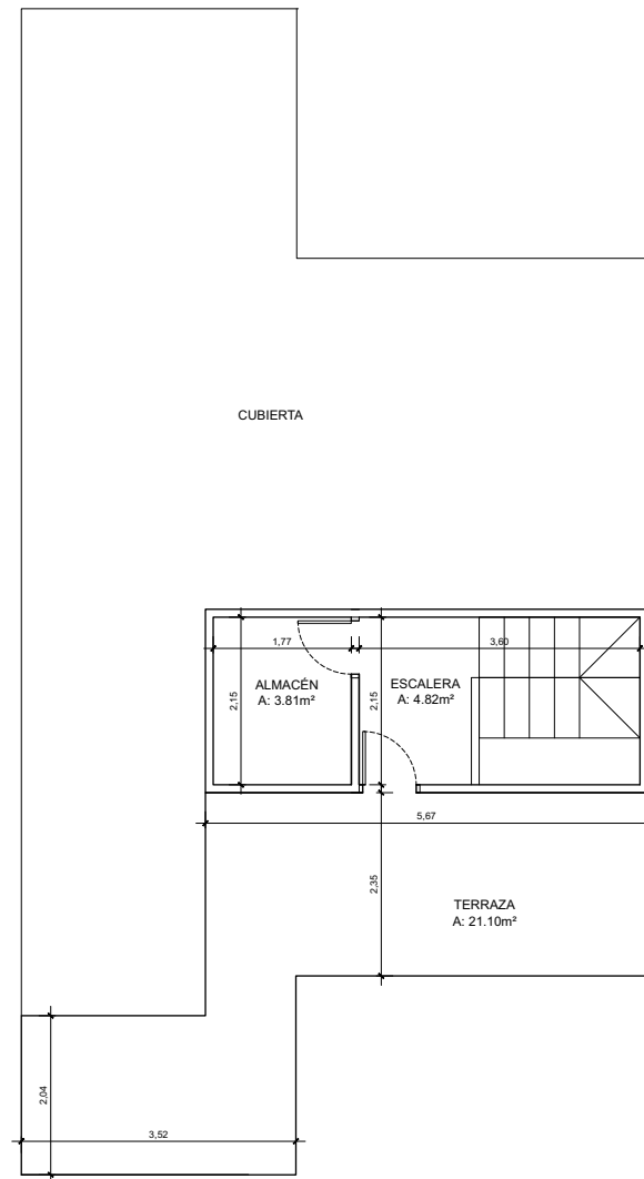
PLANTA CUBIERTA
