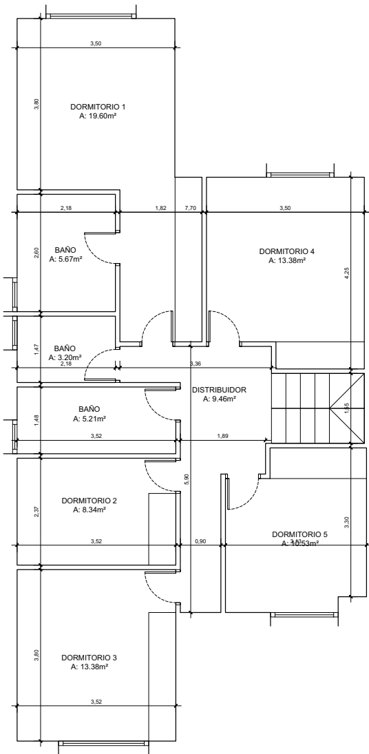
PLANTA PRIMERA
