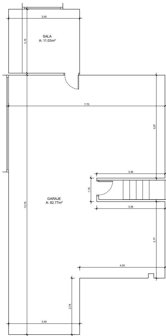
PLANTA SÓTANO
