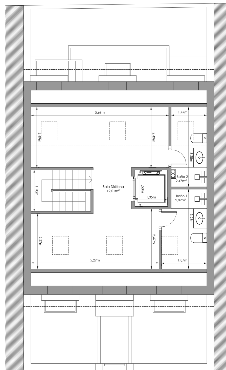
PLANTA BAJOCUBIERTA
