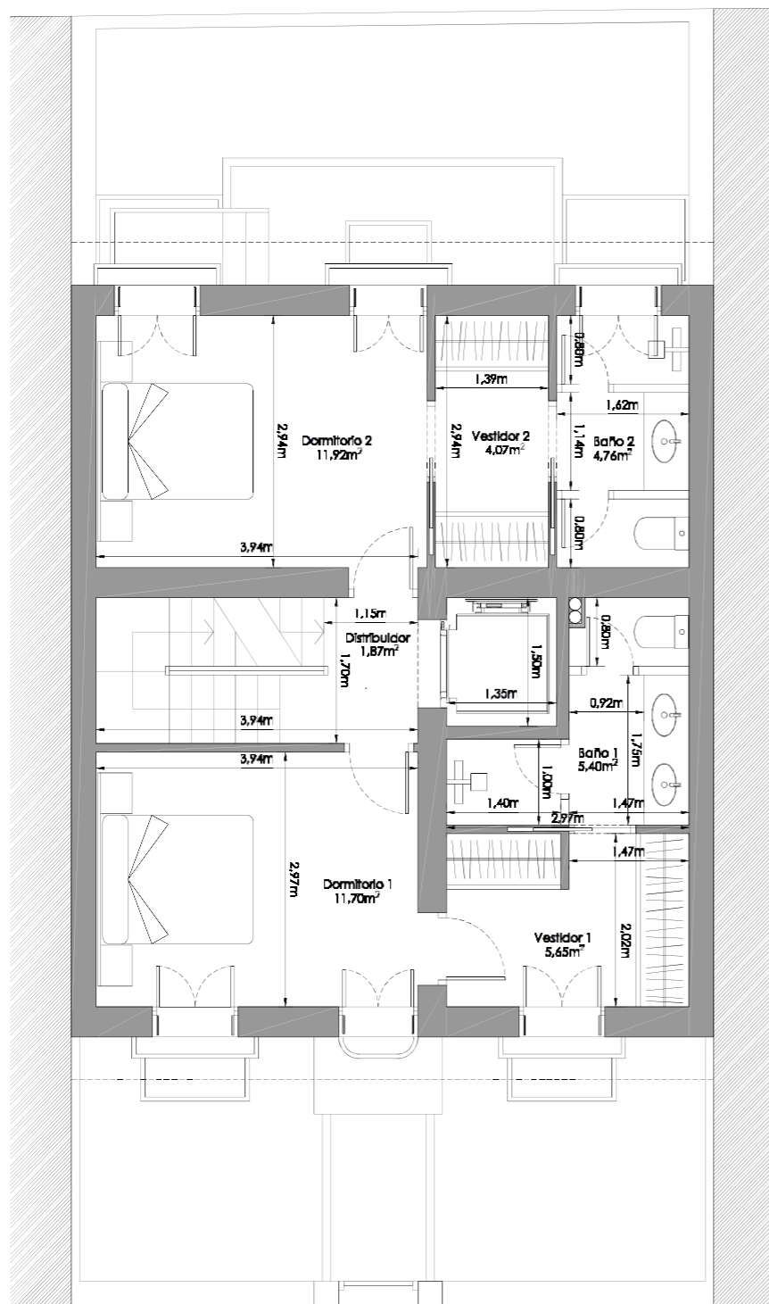
PLANTA PRIMERA
